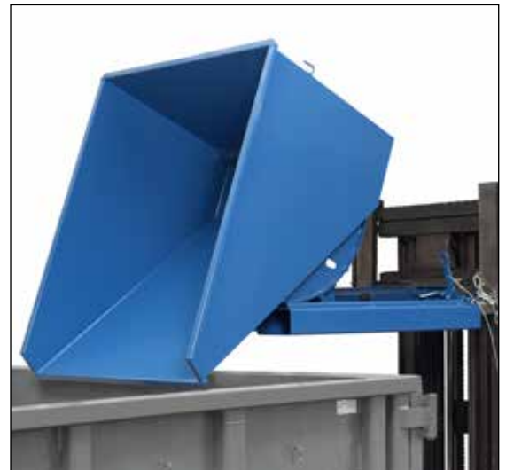
Selbstkipper als Schrotthälter mit Gabelstapler
