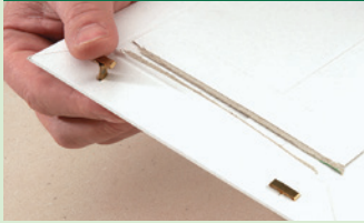
Wiederverschluss mit Clip
